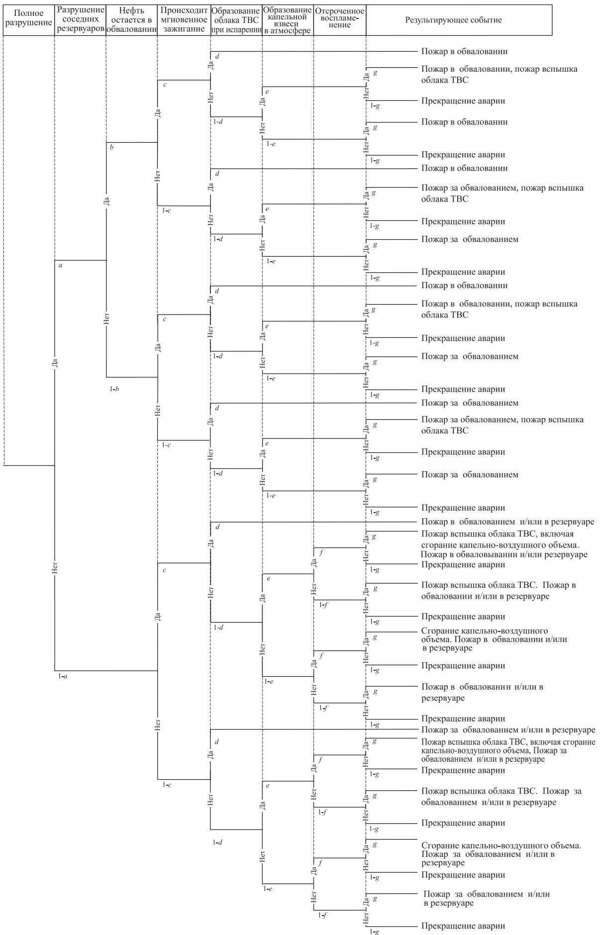
Рис. 4-1. «Дерево событий» разрушения/перелива наземного резервуара (сценарий А 1 )
