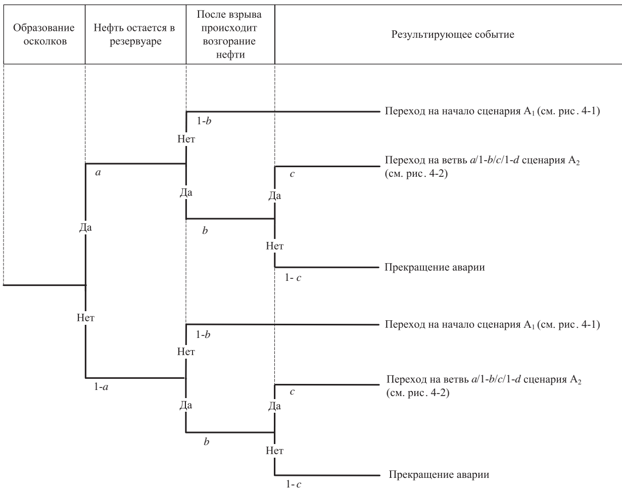
Рис. 4-3. Дерево событий при взрыве внутри наземного резервуара (сценарий A_3 )
