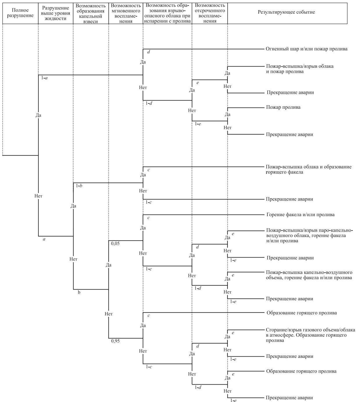
Рис. 4-7. Дерево событий при разрушении емкости под давлением (сценарий A_7 )
