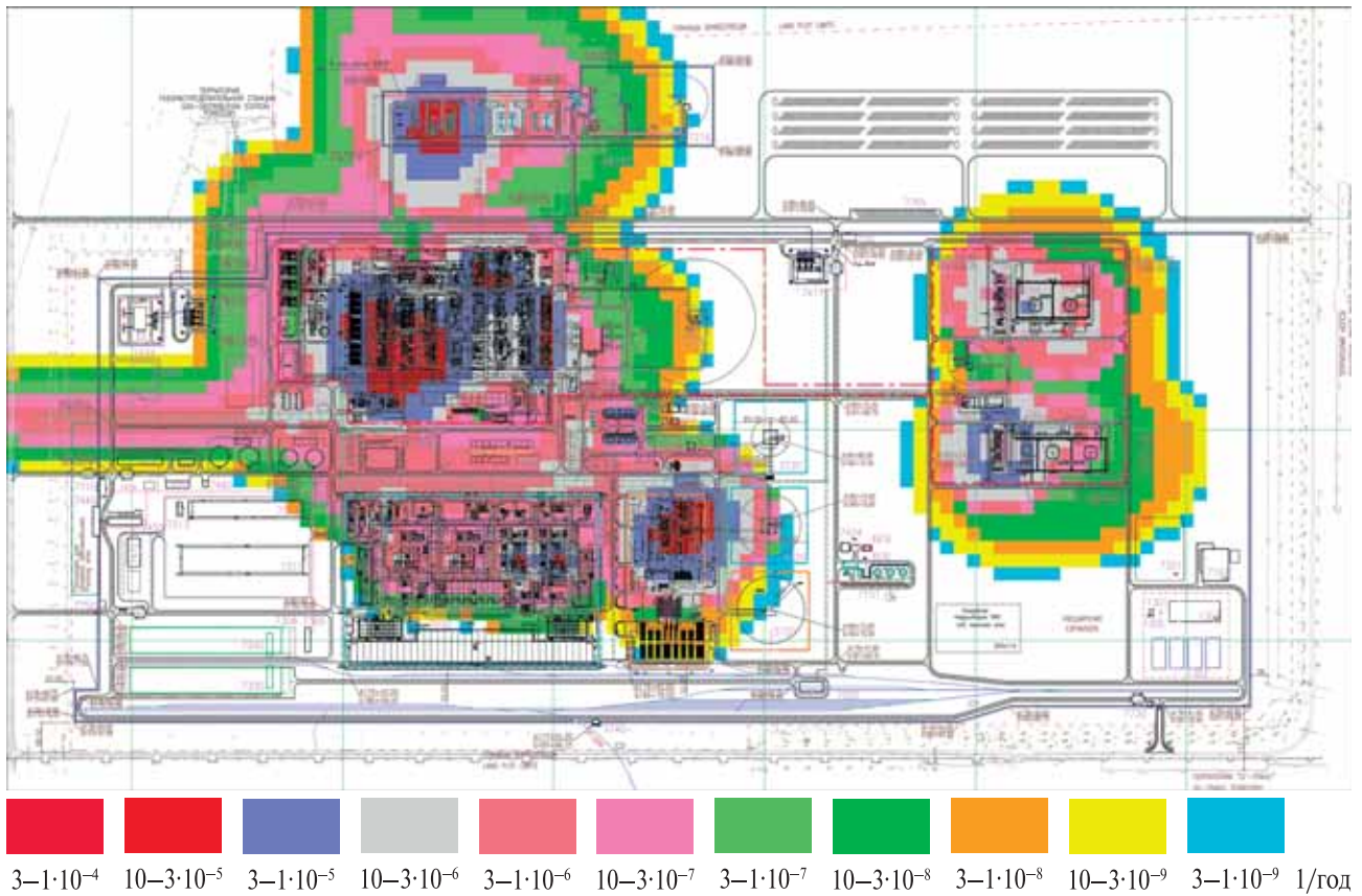
Рис. 7-2. Территориальное распределение превышения избыточного давления во фронте УВ (120 кПа) для сценариев Вво на объекте
