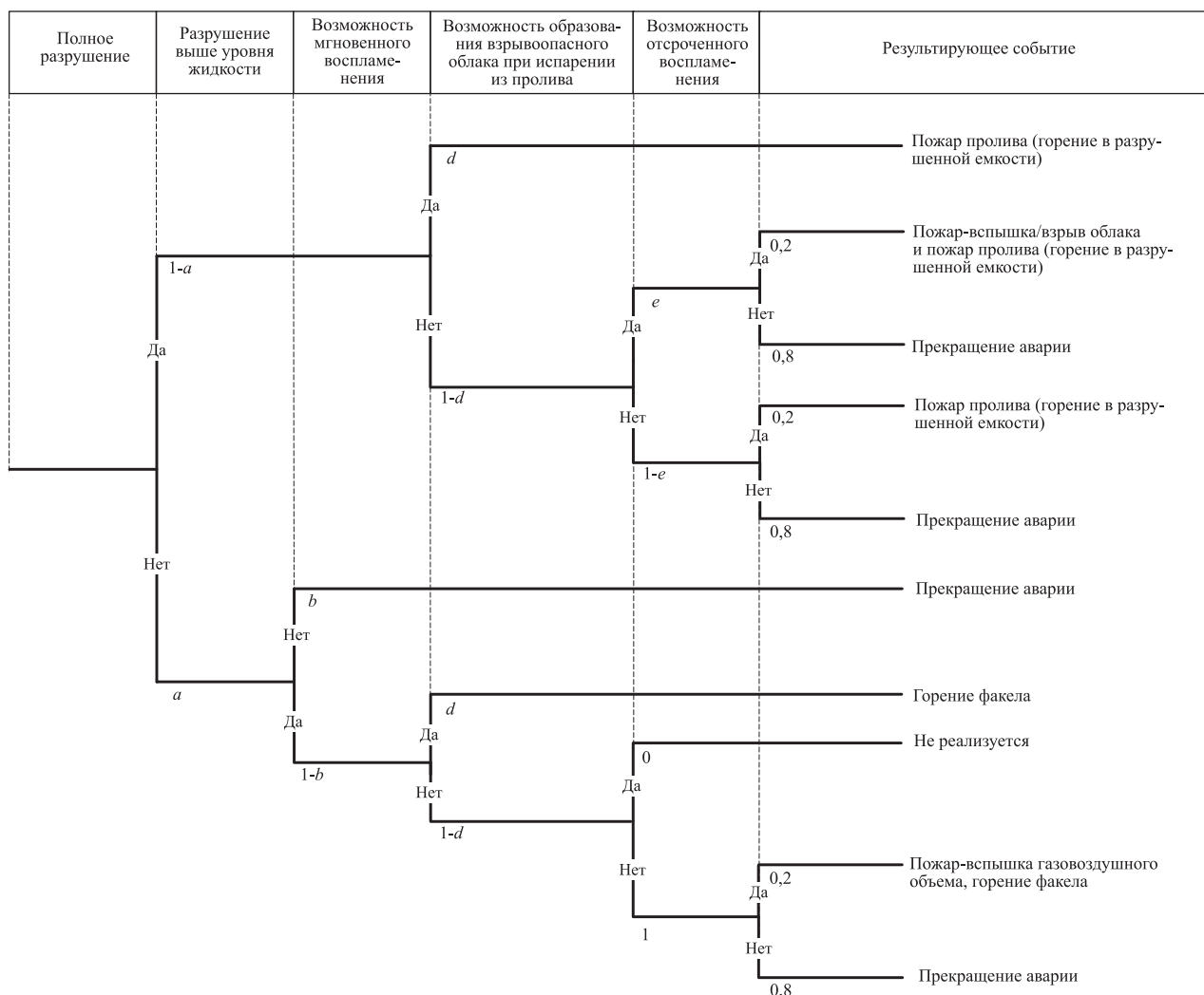
Рис. 4-8. Дерево событий при разрушении емкости под давлением (сценарий A_8 )
