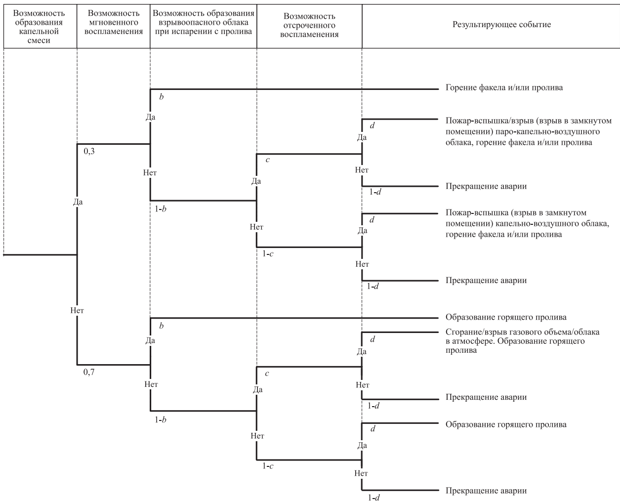
Рис. 4-9. Дерево событий при аварии в насосных (сценарий А 9 )
