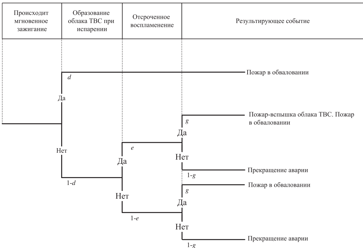
Рис. 4-4. Дерево событий разрушения/перелива подземного резервуара (сценарий A_4 )
