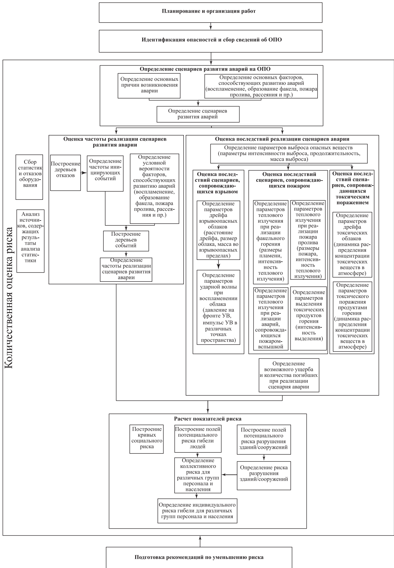
Рис. 1. Общая схема анализа опасности и оценки риска
