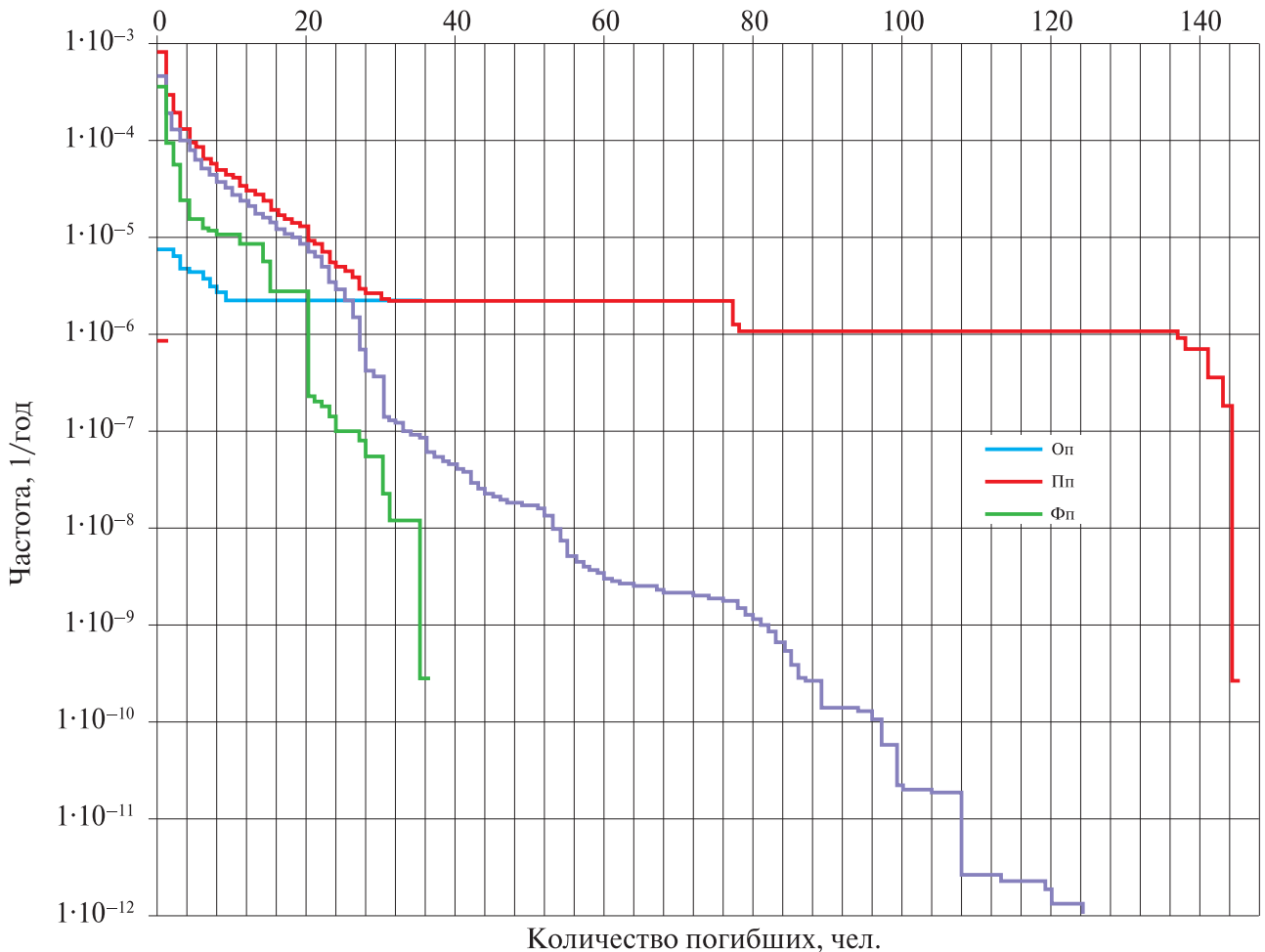
Рис. 7-1. F/N-диаграмма риска гибели людей от различных аварий на объекте
